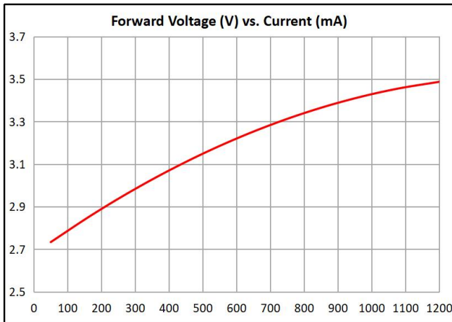
Fig 3. 正向电流 T_j=25^\circ\text{C} Forward Voltage
